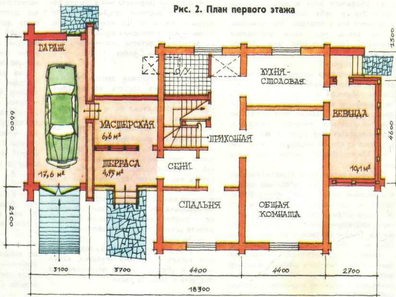
Рис. 2. План первого этажа
