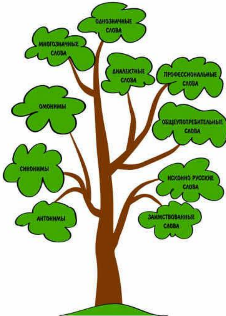
ЛЕКСИЧЕСКОЕ ДЕРЕВО
