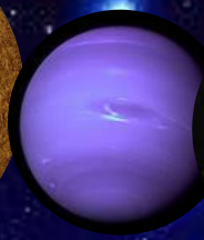
Нептун
