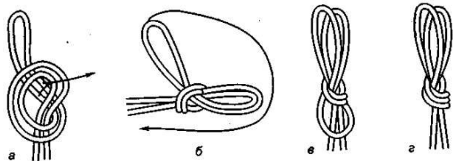
Рис. 63. «Двойной проводник»
