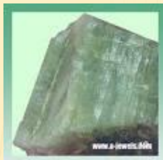
Берилл
