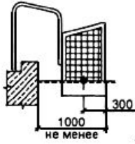
Ворота, укрепленные на торцевой стенке
