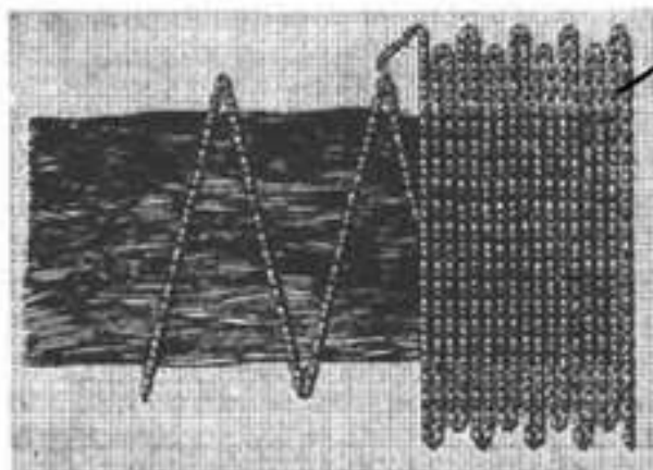
Рис. 63. Штопка по льку на швейной машинке. Наложение шва поверх пряди нитей.
