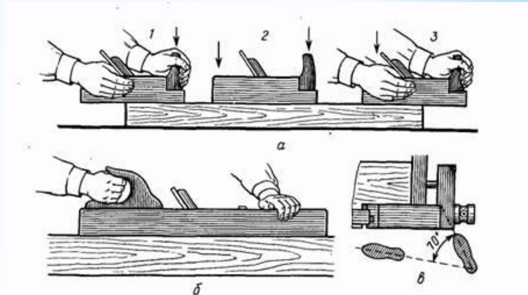
Рис. 21. Приёмы строгания:
