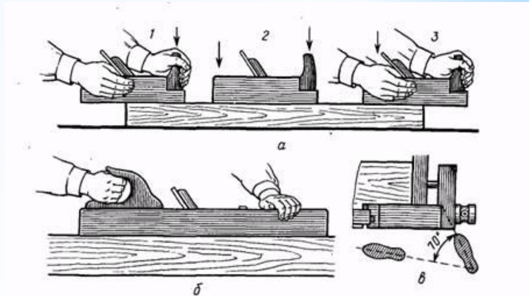
Рис. 21. Приёмы строгания:
