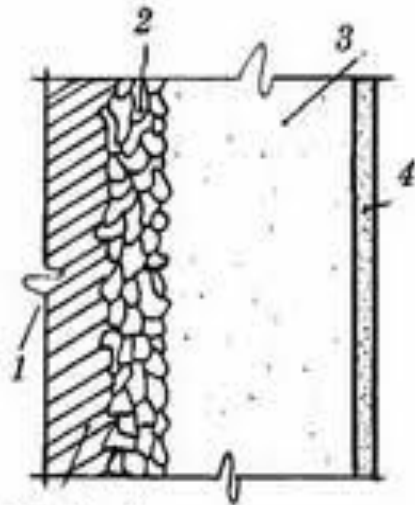
Рис. 126. Слой штукатурного намета: 1 основание-поверхность; 2 — обрызг; 3 — грунт; 4 накрывка
