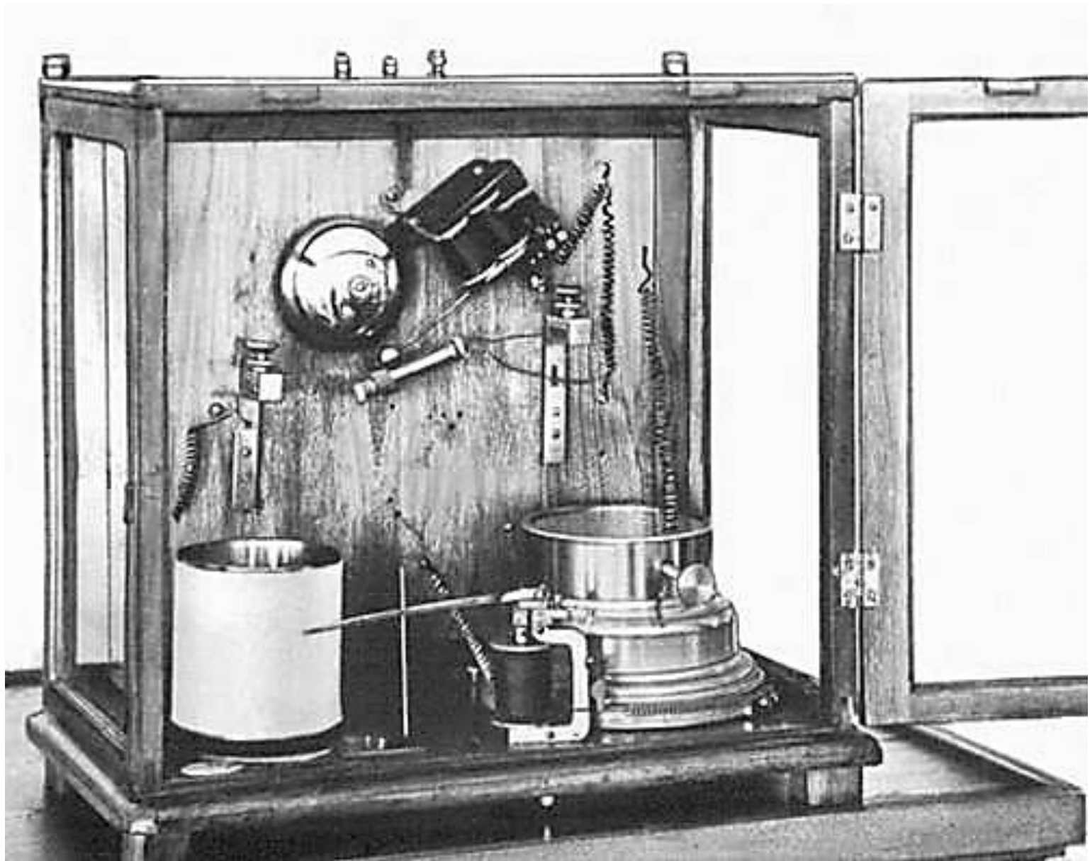
Грозоотметчик А.С. Попова
