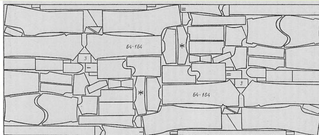
Рис. 130. Раскладка лекал деталей костюма для мальчиков из основной ткани
