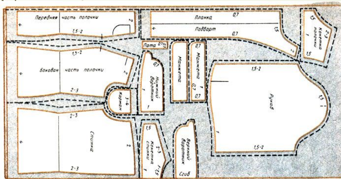
Рис. 130. Раскладка лекал деталей костюма для мальчиков из основной ткани
