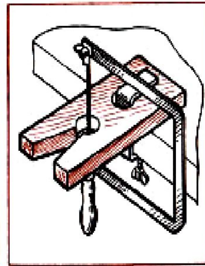
Рис. 50. Выпиловочный столик
