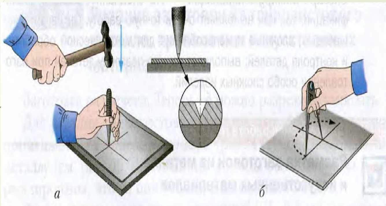
Рис. 111. Разметка окружности: a – накернивание центра окружности; б – проведение дуги
