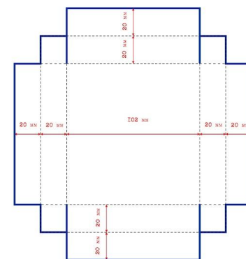
Основа крышечки
