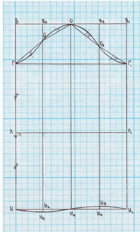
Чертеж основы рукава
