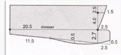
Чертеж воротника на стойке
