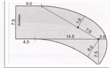
чертеж круглого плоского воротника
