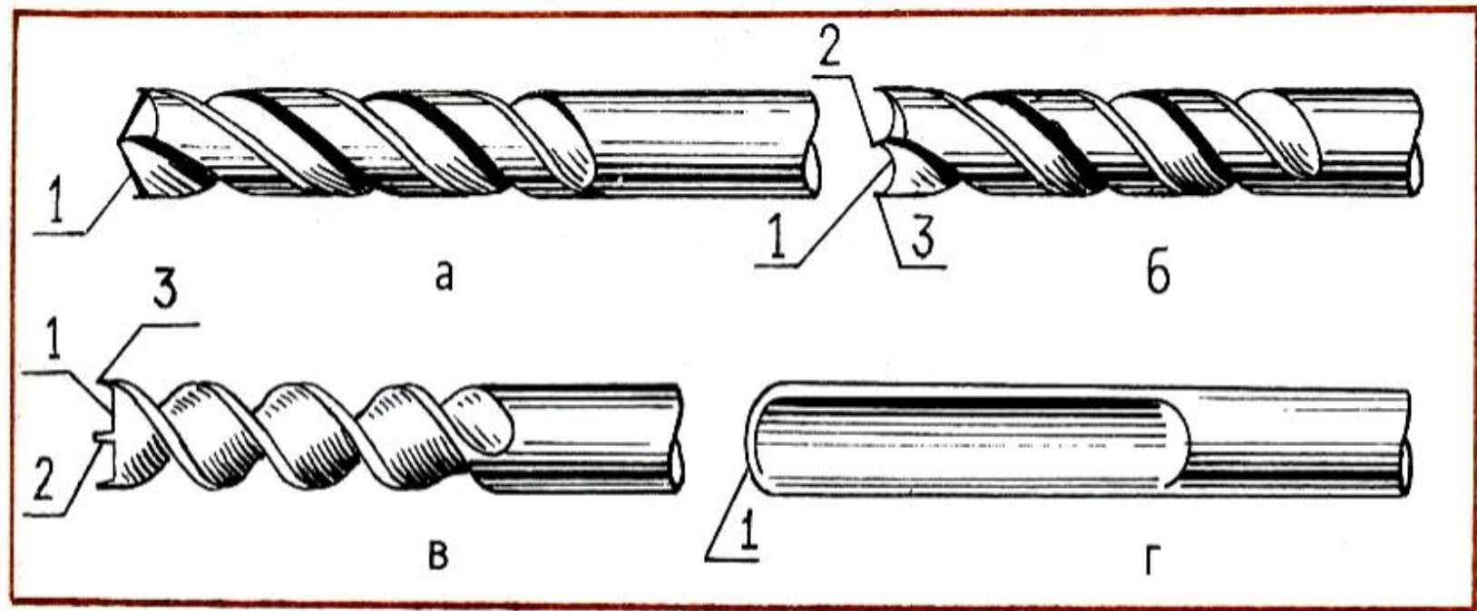
Рис. 34. Сверла:
