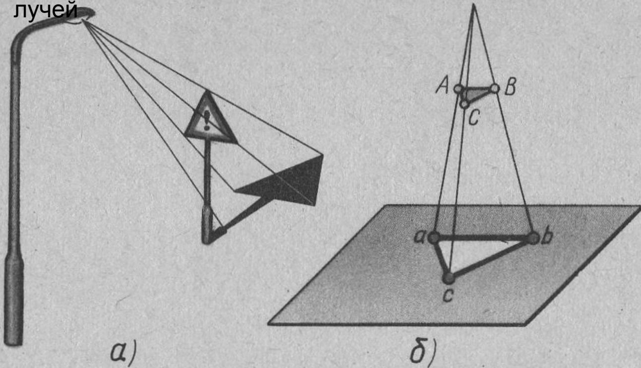
Рис. 33. Центральное проектирование
