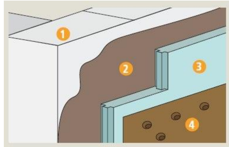
Схема гідроізоляції фундаментної стіни
