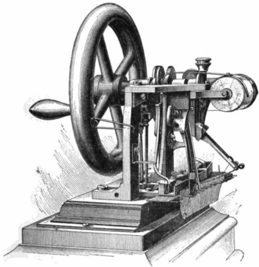
Elias Howe's lockstitch machine, invented 1845/Швейная машина изобретённая Элиасом Хоу в 1845 г.
