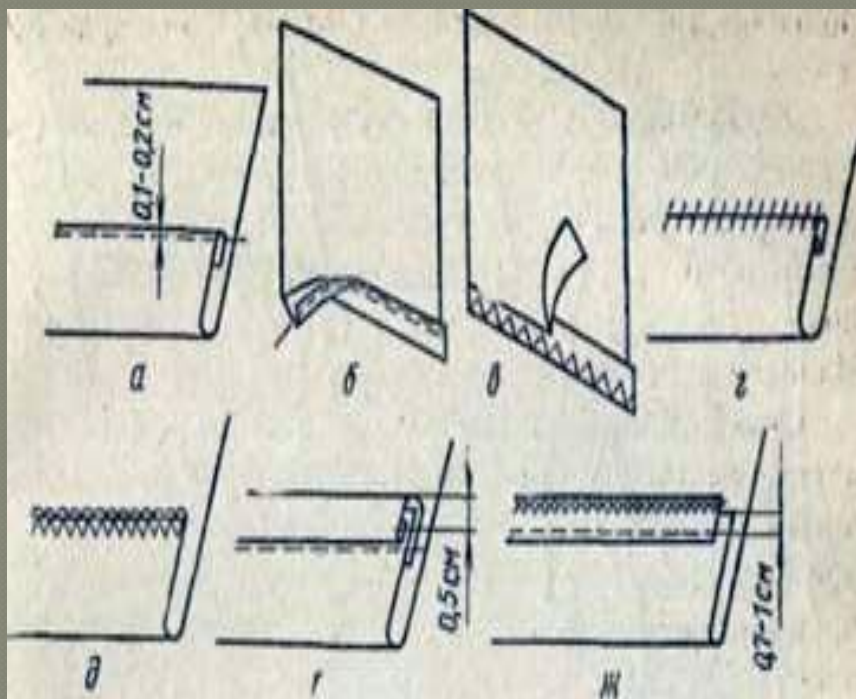
Рис. 87. Обработка низа изделий
