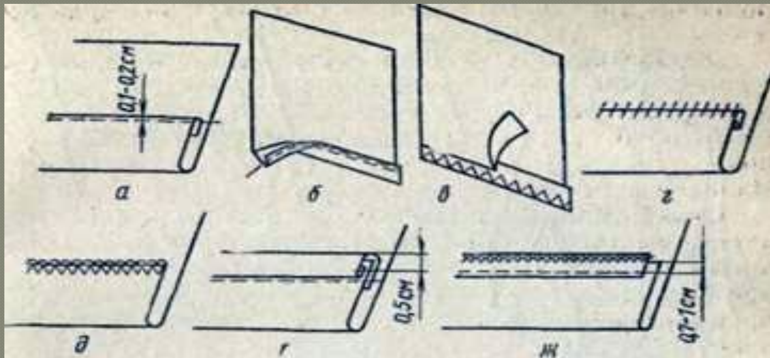
Рис. 87. Обработка низа изделий
