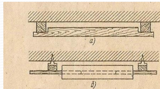
Рис. 42. Установка деревянных маяков:
