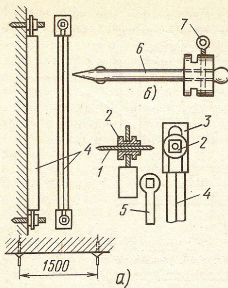
Рис. 47. Инвентарные металлические маяки: a — маяк и его детали, б — конструкции штыря и гайки: 1, 6 — штыри, 2 — гайка, 3 — косынка, 4 — уголок, 5 — ключ, 7 — винт
