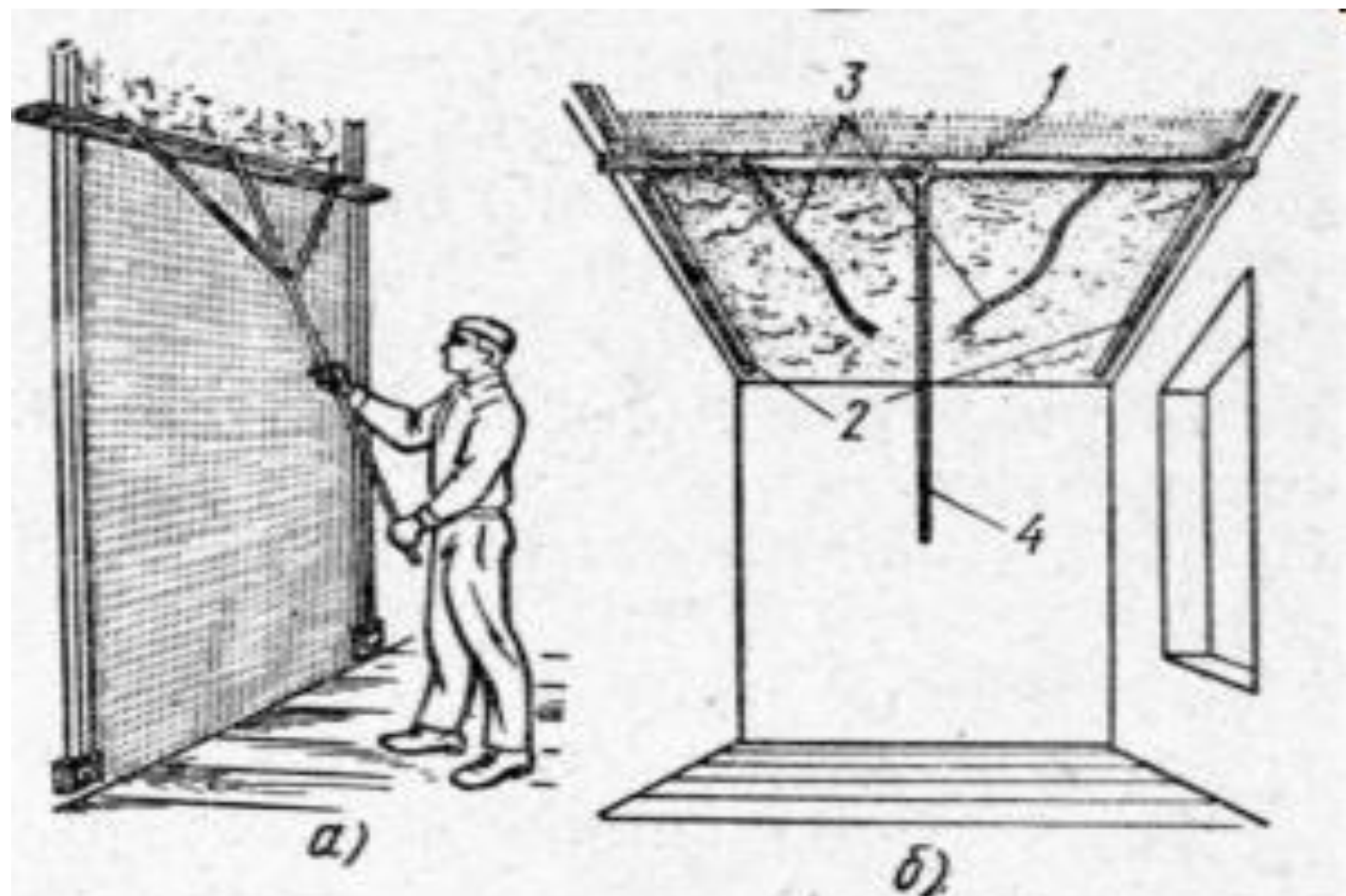
Рис. 49. Разравнивание раствора: а — правилом на ручке на стенах по металлическим маякам, б — малкой на потолках; 1 — малка, 2 — маяки, 3 — веревки, 4 — держало
