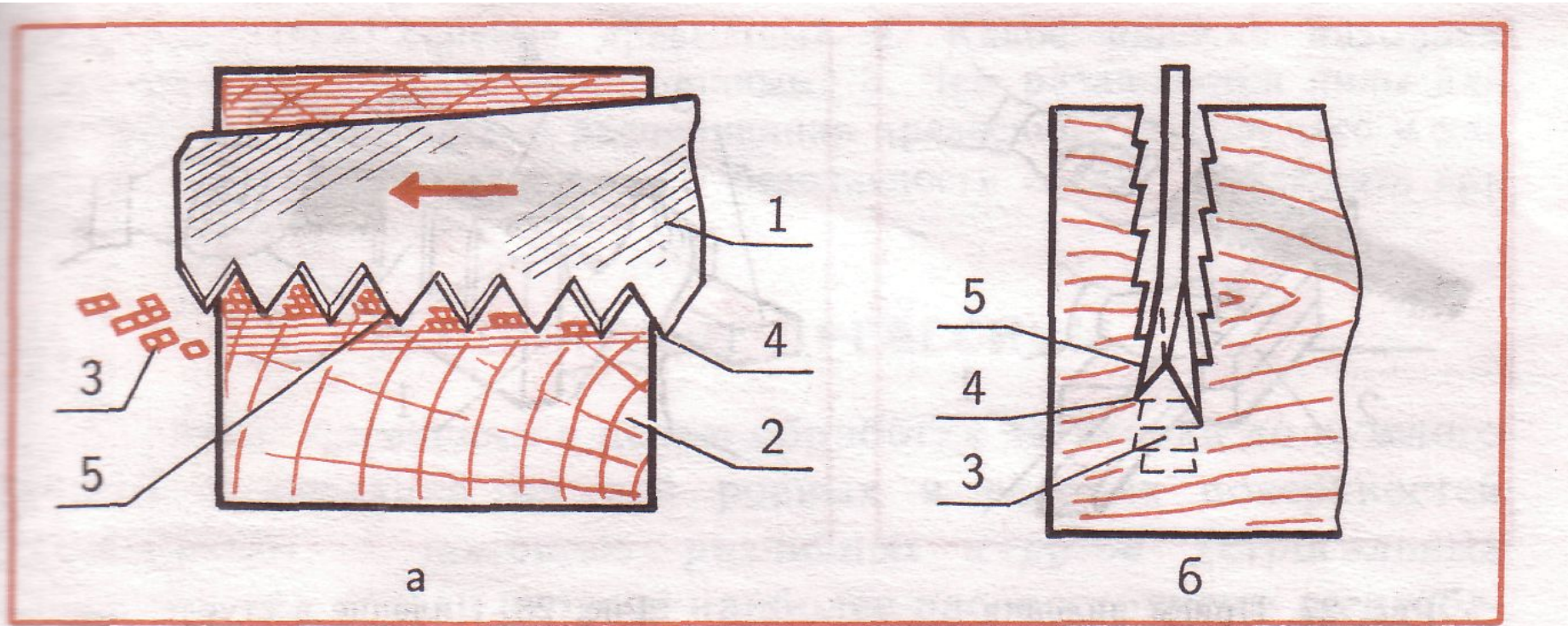
Рис. 25. Поперечное пиление:
