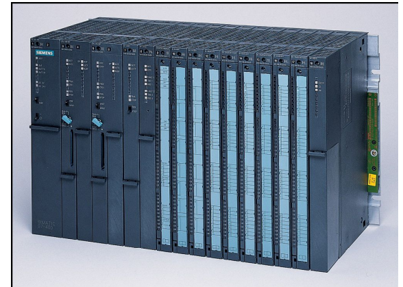
Контроллер SIMATIC S7- 400 компании SIEMENS
