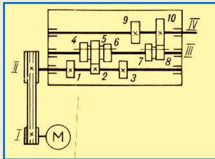
Кинематическая схема
