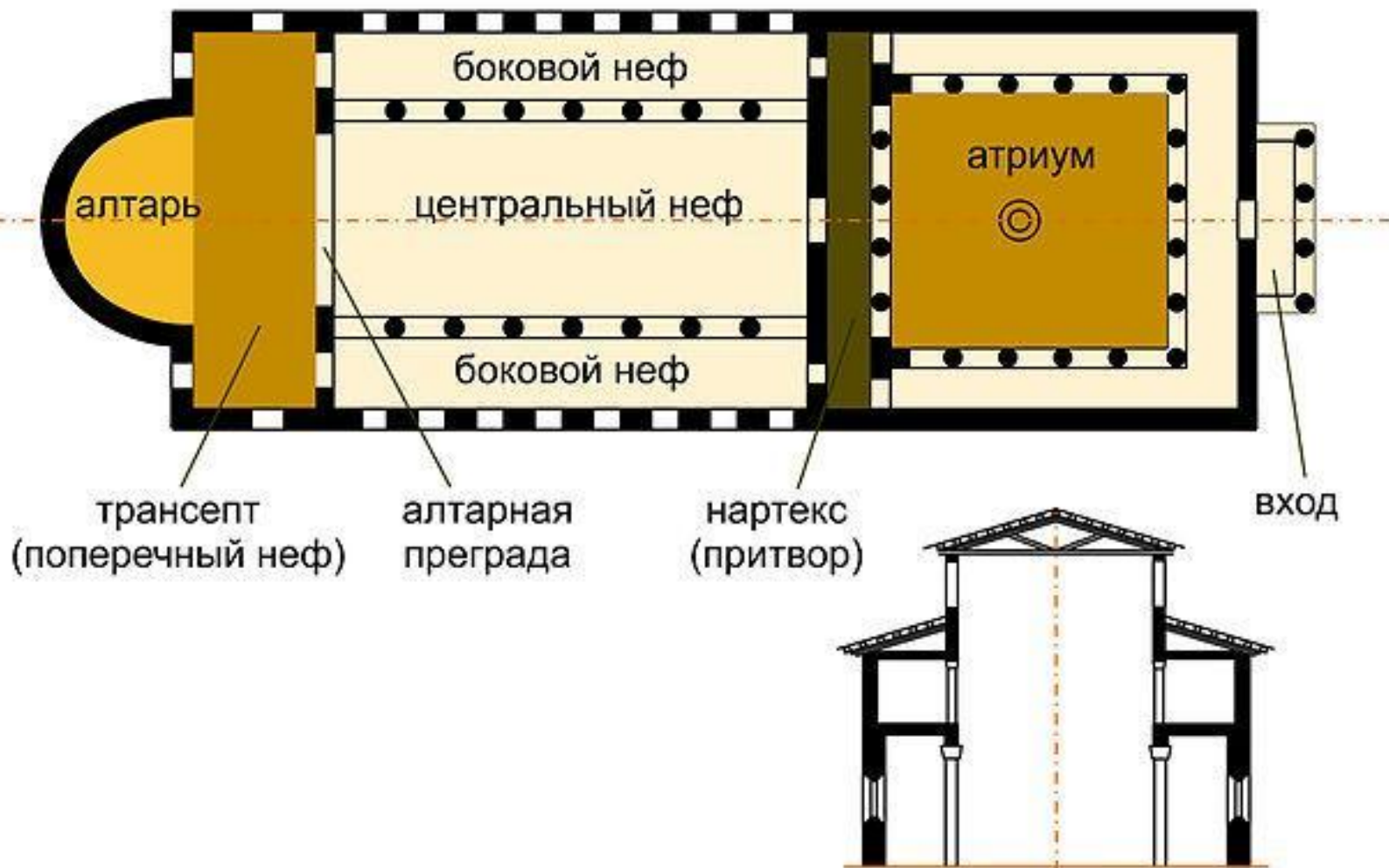
План и конструкция христианской базилики
