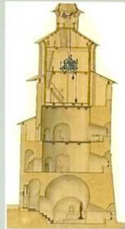
Этаж-проектирование Башни над Часик № 11. Разрез. 1879 г.
