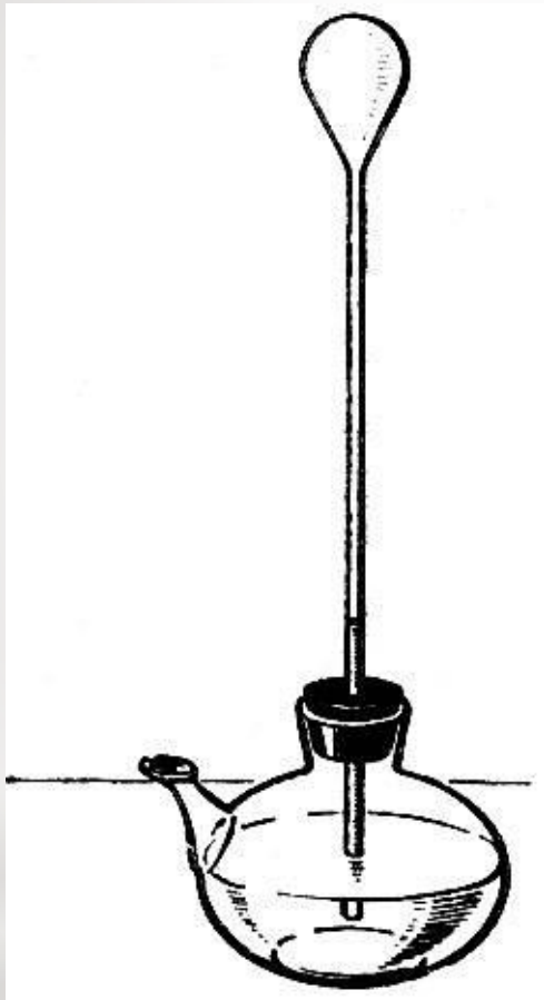
Термоскоп
