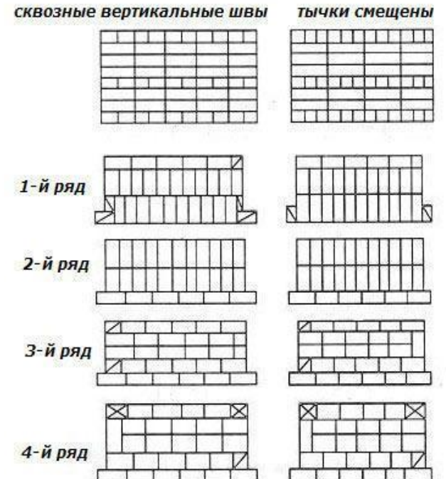
Декоративная лицевая кладка с неперевязанными вертикальными швами
