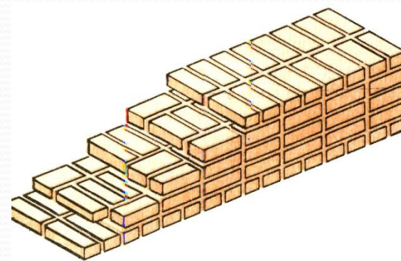
Перевязка кладки при декоративном рисунке на лицевой поверхности
