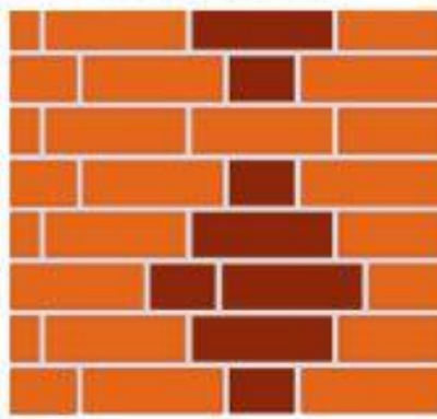
бранденбургская модифицированная
