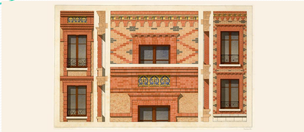
Кладка стены с декоративным рисунком швов
