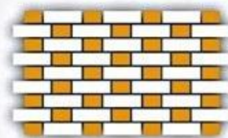
Фламандская кладка
