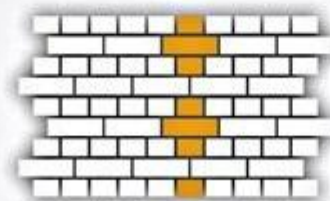
Крестовая кладка
