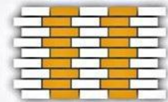
Ложковая кладка смещение на 1/4 кирпича
