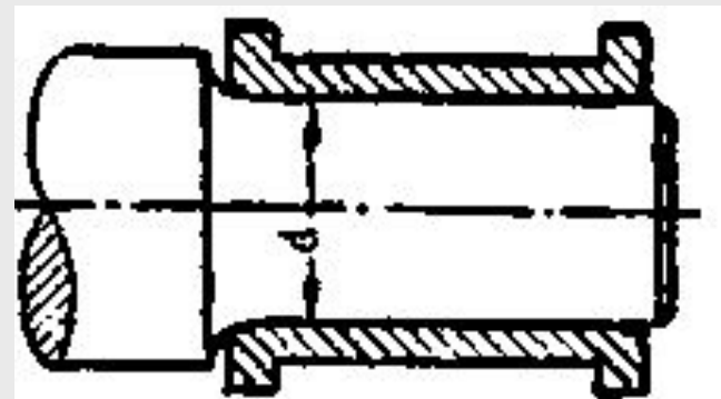
Подшипник скольжения из антифрикционного чугуна
