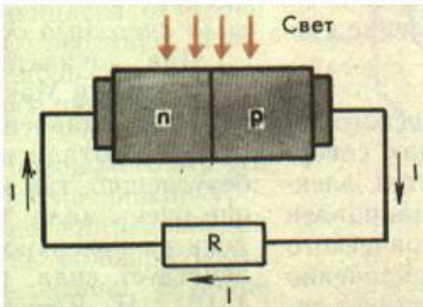
Полупроводниковые фотоэлементы.
