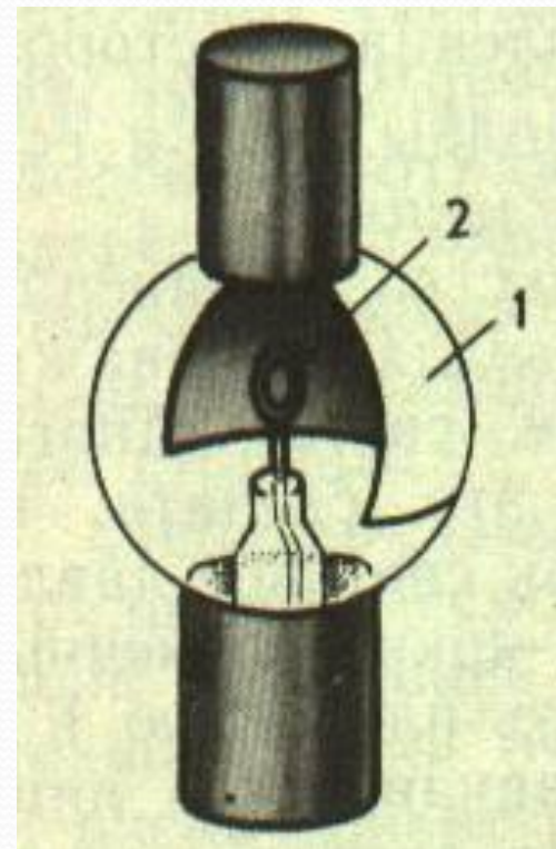
Вакуумные фотоэлементы.
