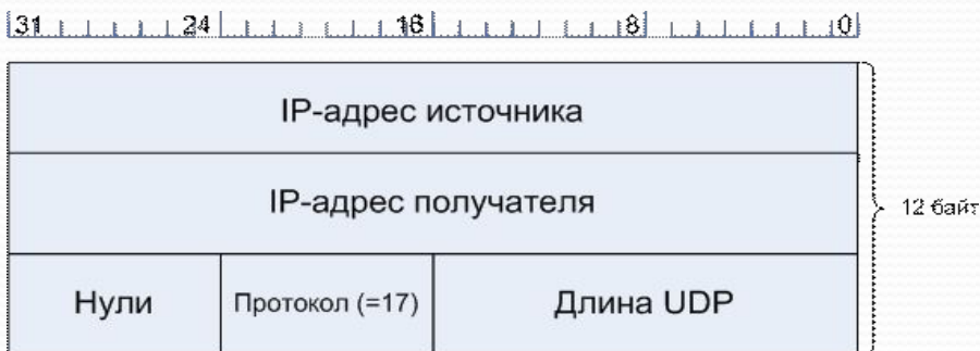
Рис. Структура псевдозаголовка пакета UDP
