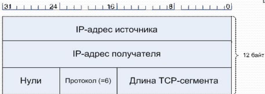
Рис. Структура псевдозаголовка пакета TCP.
