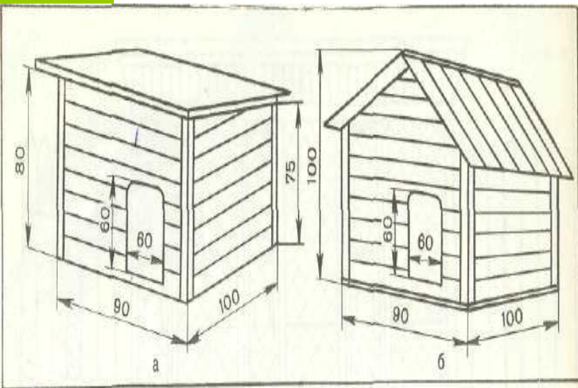
Будки для содержания собак: А-односкатная; Б- двускатная (размеры даны в сантиметрах)
