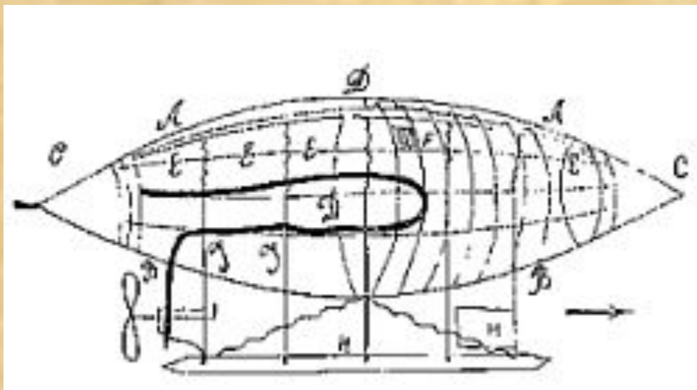
Чертеж проволочной модели дирижабля Циолковского
