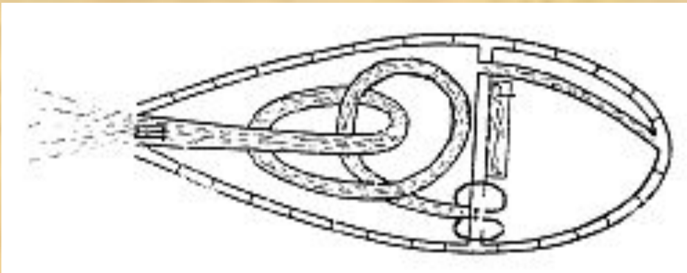
Ракета К.Э. Циолковского. 1914г.
