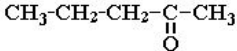
пентанон-2
