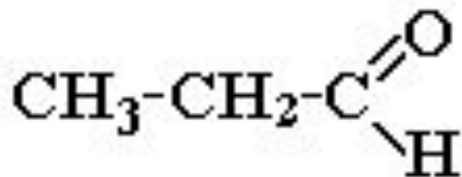
пропаналь
