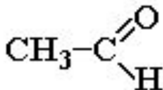
этаналь (ацетальдегид)
