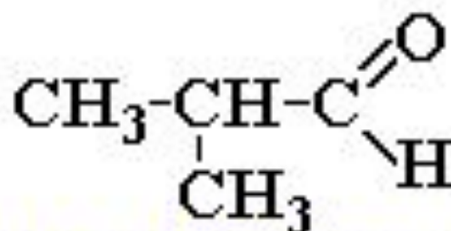
2-метилпропаналь
