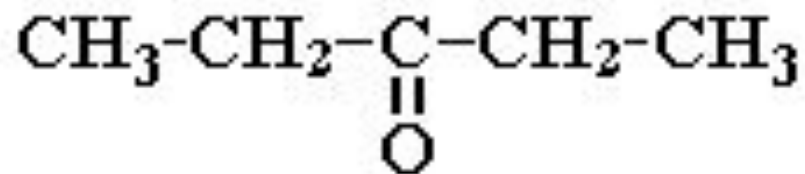
пентанон-3
