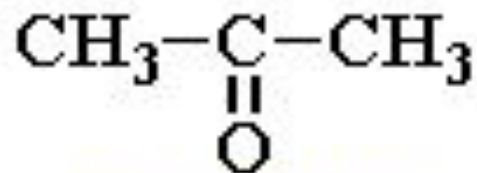
пропанон (ацетон)
