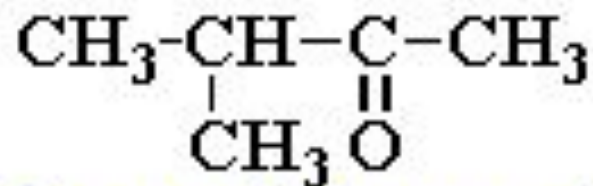
3-метилбутанон-2
