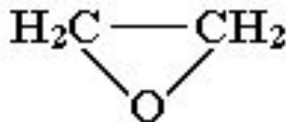
этиленоксид
