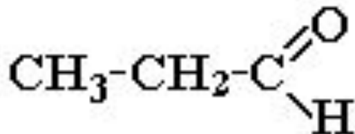
пропаналь
