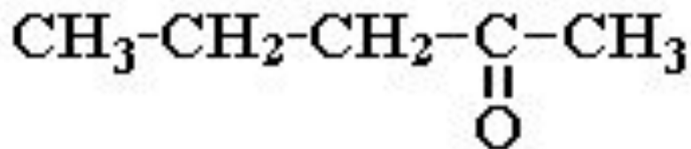
пентанон-2
