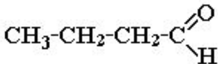
бутаналь
