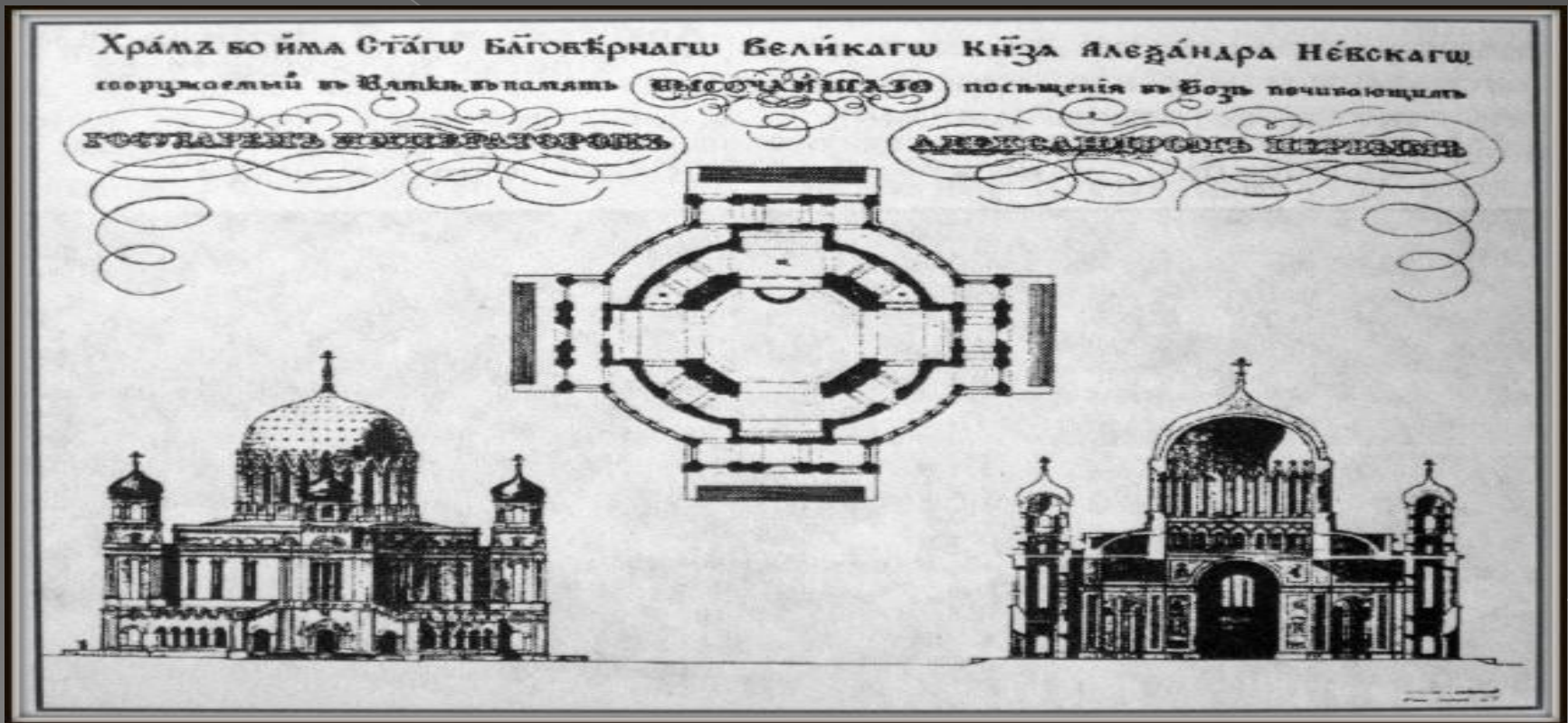
Алекса́ндро-Невский собор. План (вид сверху), фасад и боковой разрез.
