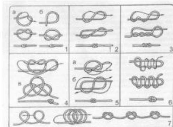
Рис. 1. Узлы для утолщения троса: 1 — «простой»; 2 — «восьмерка»; 3 — «стаканчик»; 4 — «куриный»; 5 — «юферный»; 6 — «многократная восьмерка»; 7 — «пожарная лестница»; а, б — варианты вязки; в — узел-орнамент
