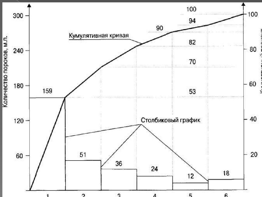
Рис 1. Диаграмма Парето по видам дефектов: 1 — концевые; 2 — складки; 3 — засечки; 4 — вмятины; 5 — грязь; 6 — прочие
