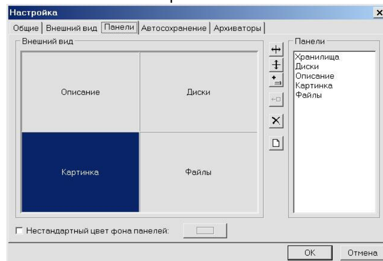
Настройка панелей
