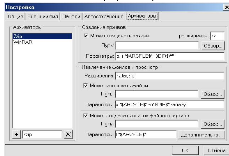
Выбор архиваторов
