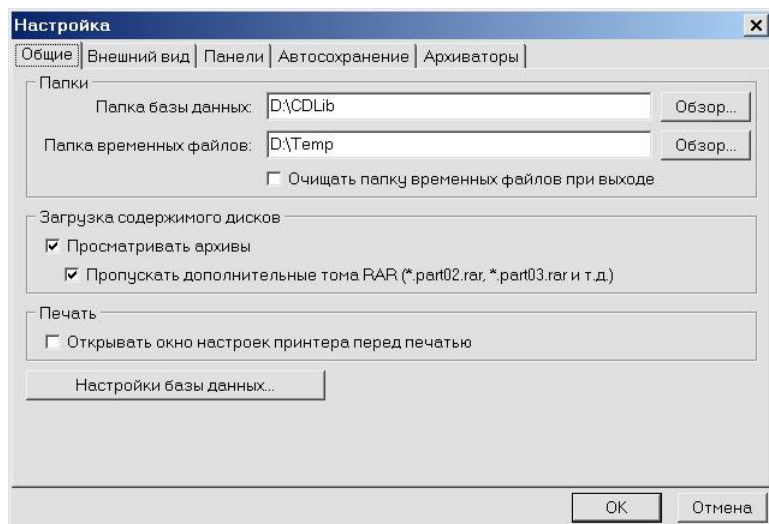
Общая настройка
