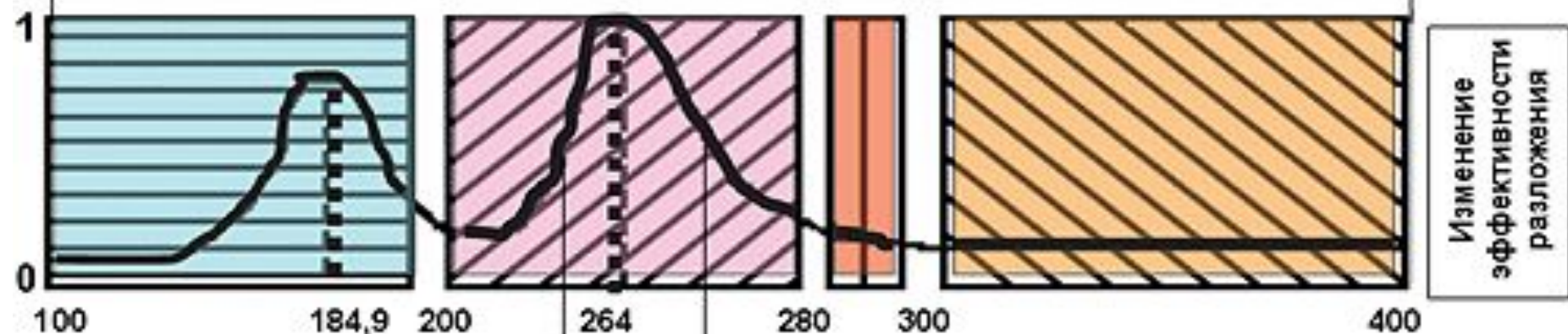
Спектр ультрафиолетового излучения лампы «BioZone»
