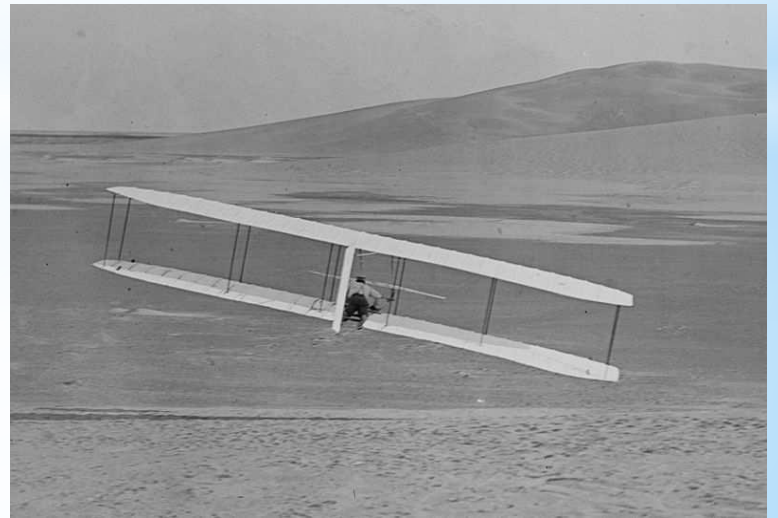
* Планер 1902 г
