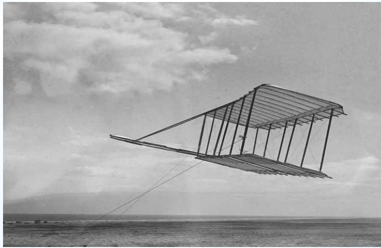
* Планер 1900 г (маленькая подъемная сила)
