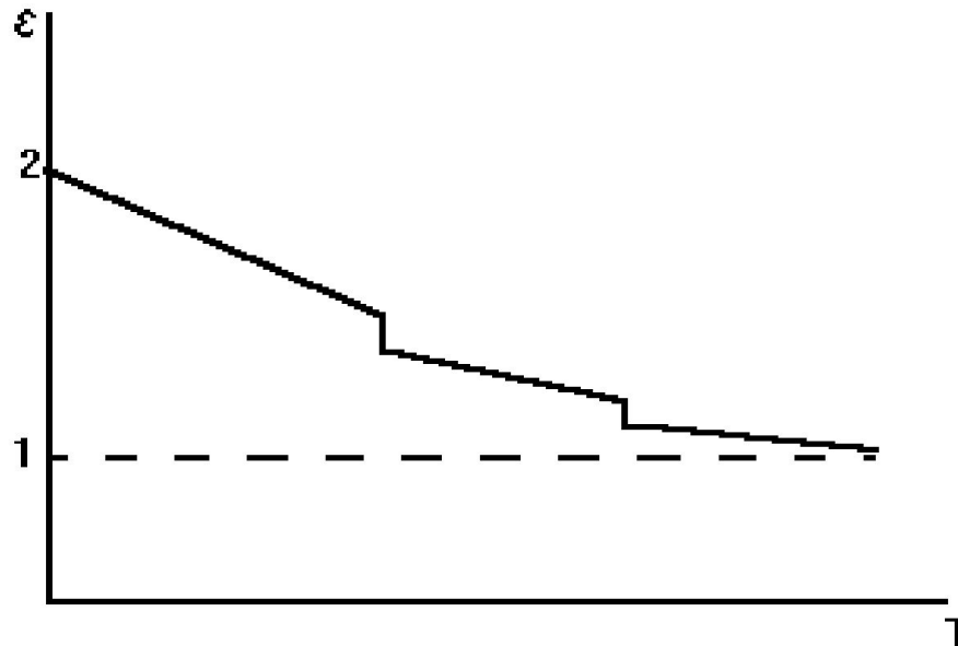
Рис. 3. Зависимость диэлектрической проницаемости от температуры для неполярных диэлектриков.
