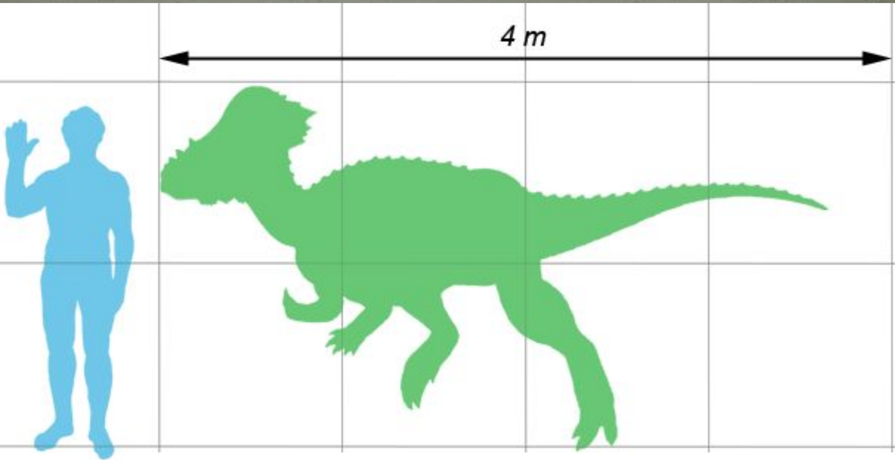
Pachycephalosaurius wyomingensis
