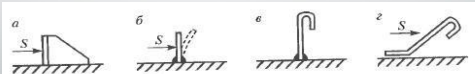
Рис. 5.3. Принципиальные типы упоров: a — жесткий; б — гибкий штыревой; в — вертикальный анкер; г — наклонный анкер
