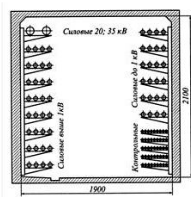
Прокладка кабелей в туннеле
