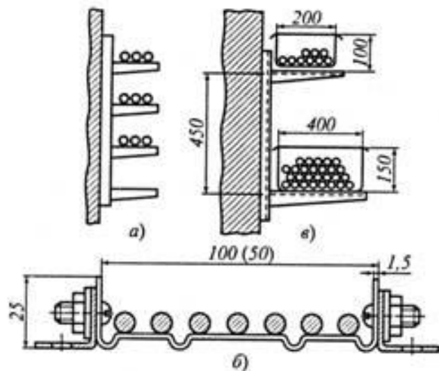
Прокладка кабелей
