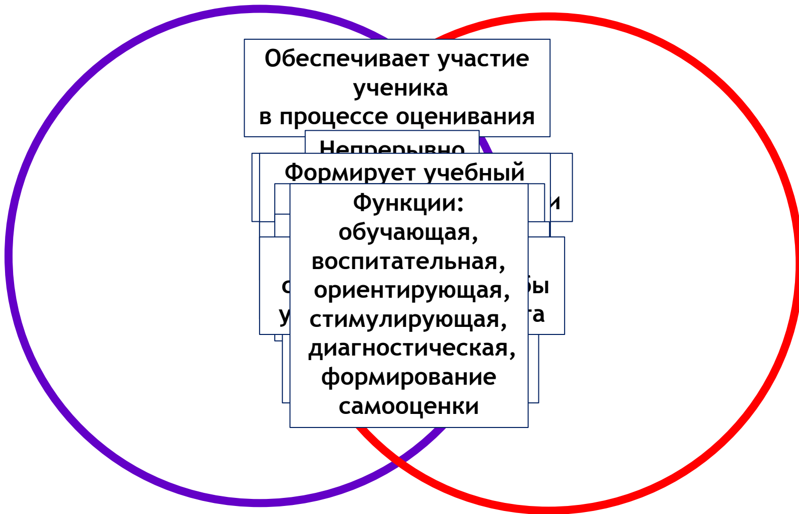
ДИАГРАММА ВЕННА
