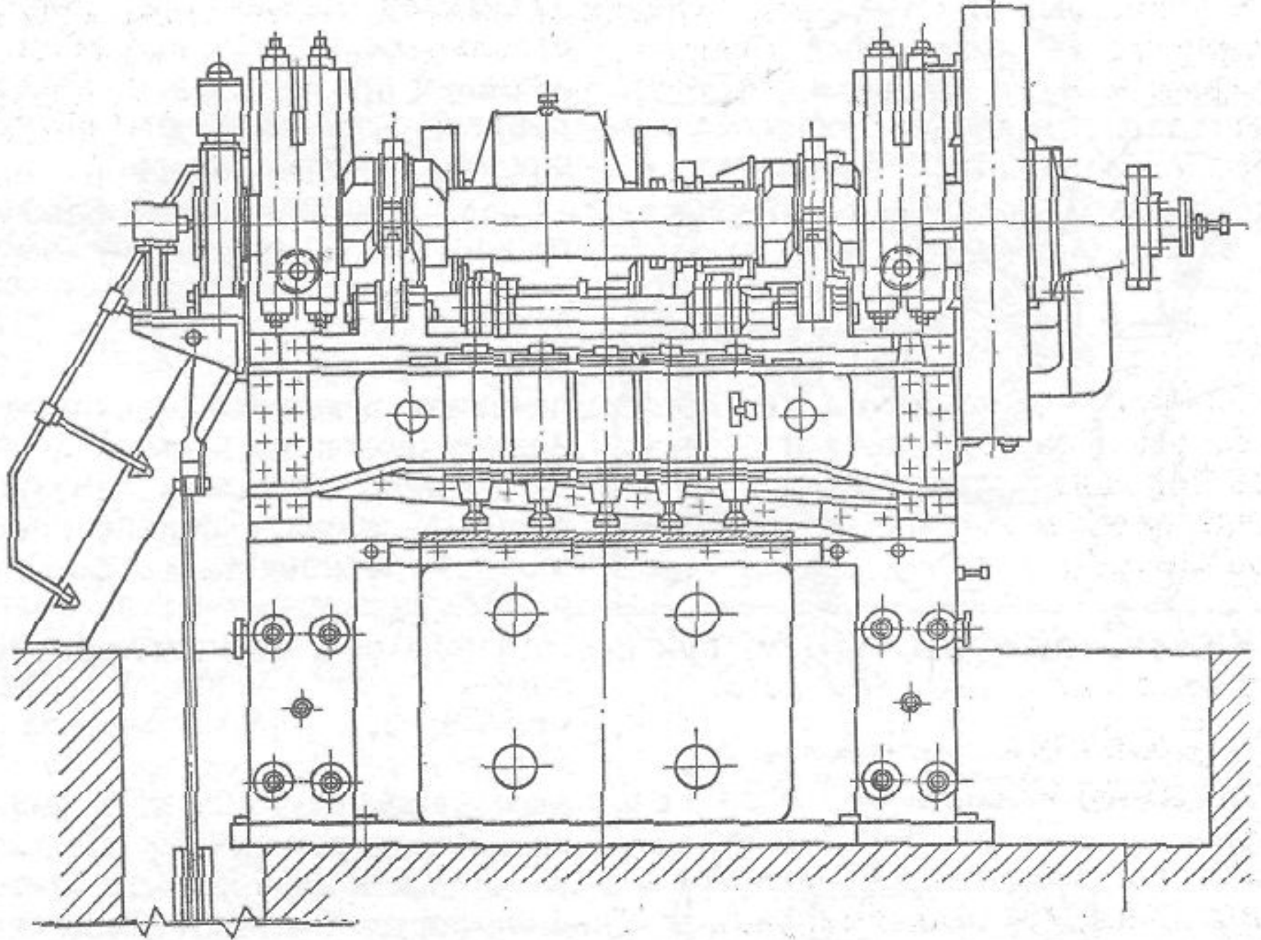
Гильотинные ножницы с верхним резом.
