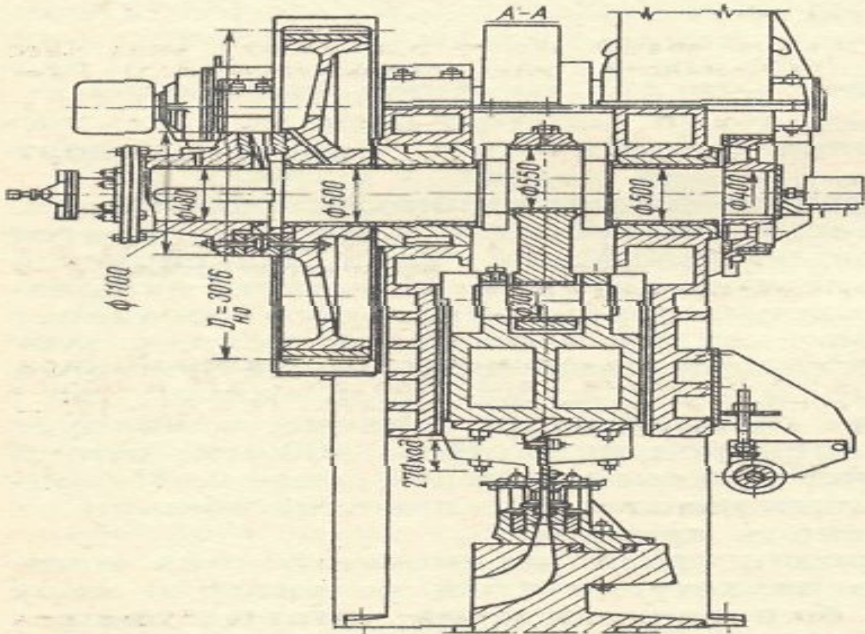
Сортовые гильотинные ножницы открытого типа
