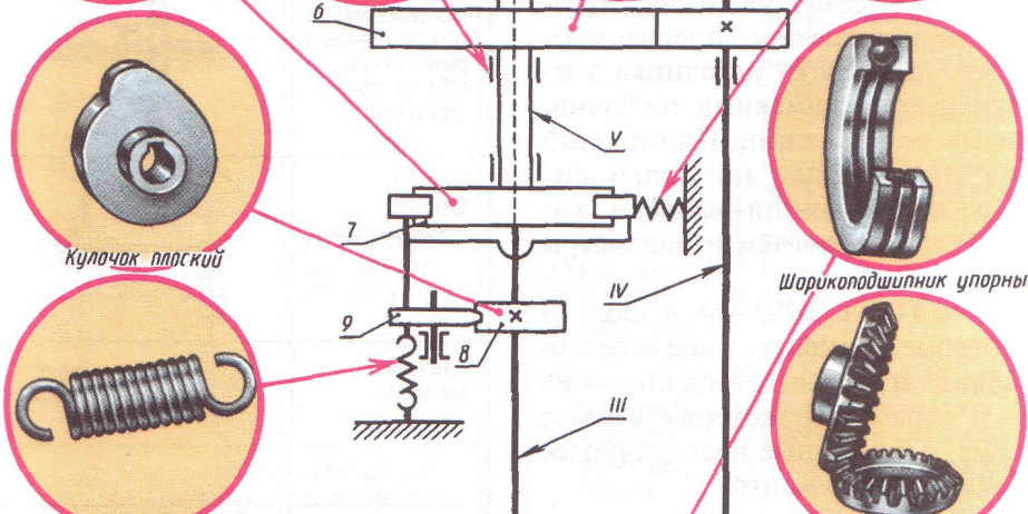
Пружина растяжения
