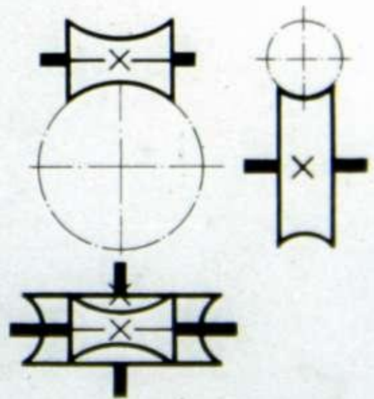
Глобоидная
