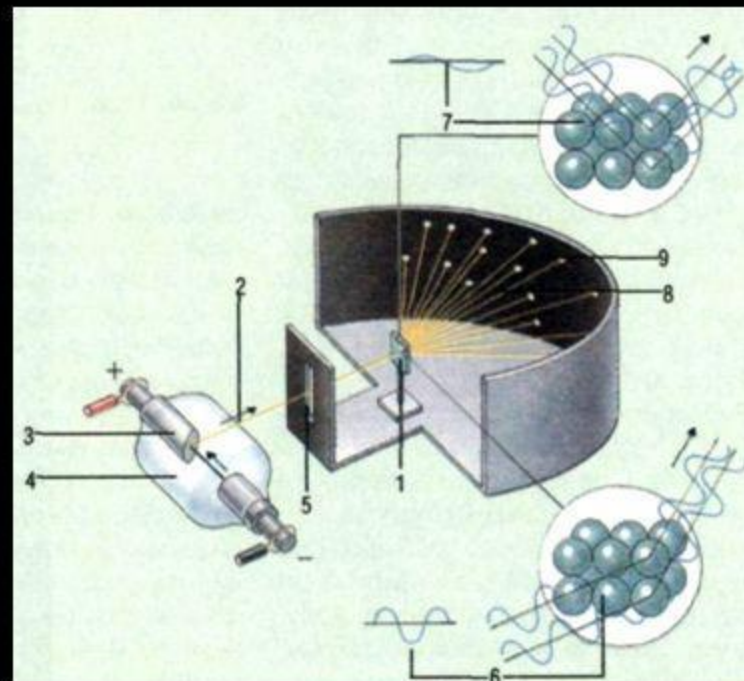
рентгеноструктурный анализ
