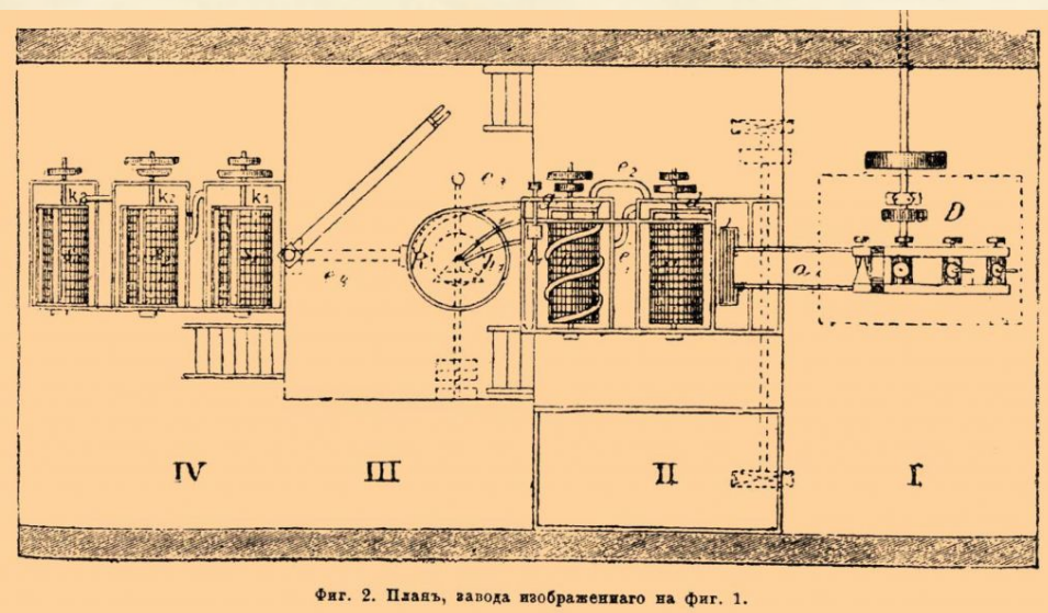
Фиг. 2. Планъ, завода изображеннаго на Фиг. 1.
